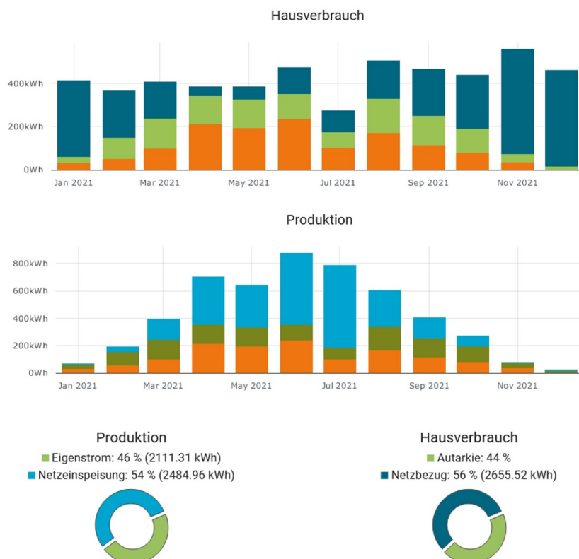
Abbildung 46: Stromproduktion und -verbrauch eines Einfamilienhauses (4 Personen) mit einer 6,9 kWp-PV-Anlage und 6 kW Speicher(Quelle: Zeiten°Grad)
